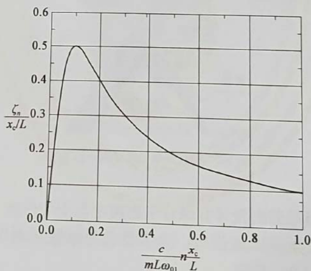
图 9-6 通用阻尼器设计曲线
