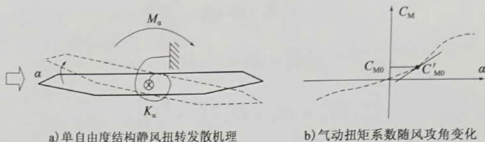
图 7-2 静风扭转发散机理示意图
