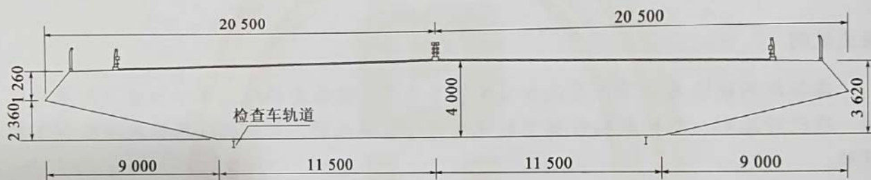
图 D-1 断面布置尺寸图 (尺寸单位: mm)
