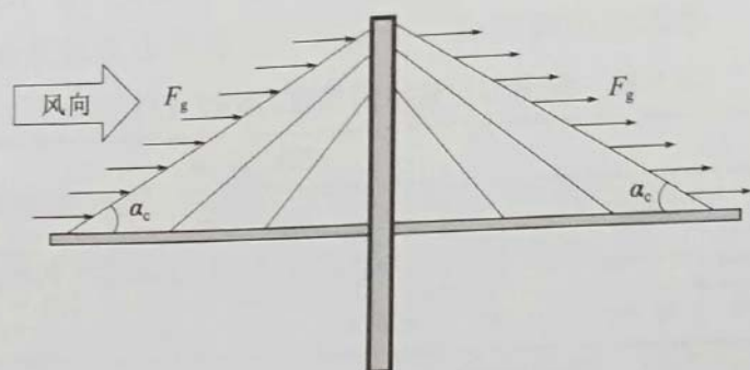
图 5-14 斜拉索倾斜角定义示意图
