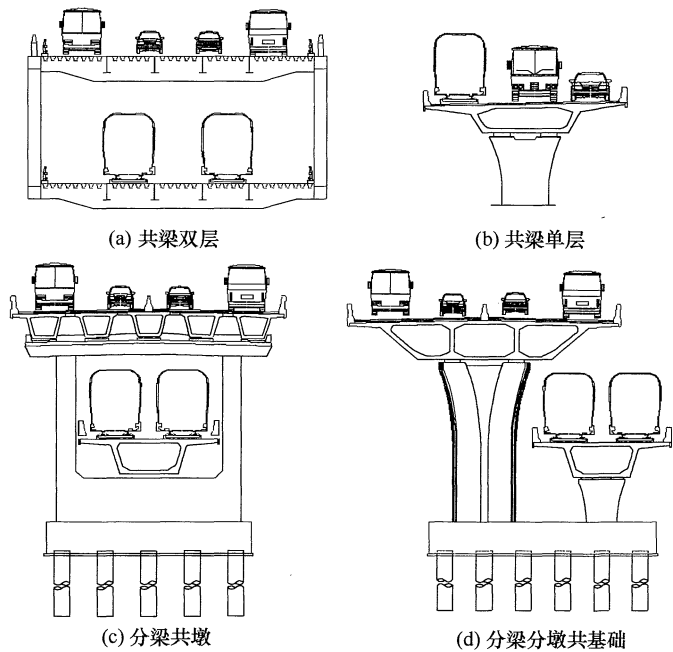
图 1 合建桥梁交通布置示意
