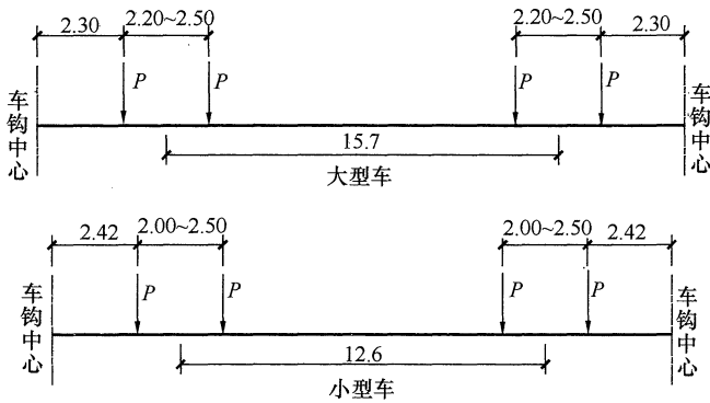
图 5 单列车静活载计算图式（尺寸单位以米计）
